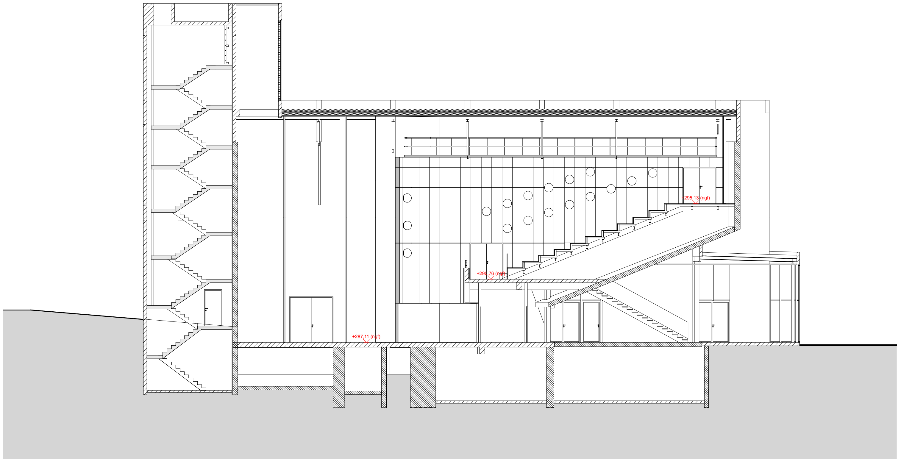
coupe sur gradins au droit du mur côté cour
